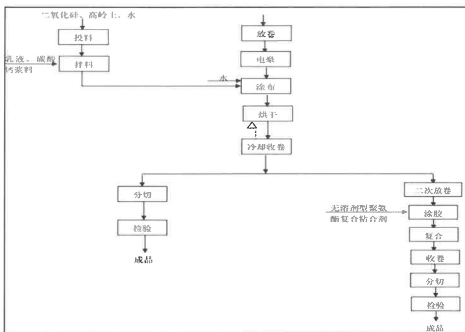
图 2 产品生产工艺流程图
